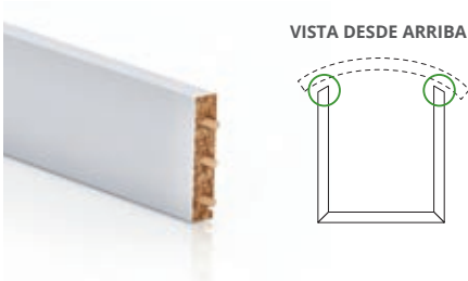
ESCUADRADO INCLINADO PARA FRENTE CURVOS
